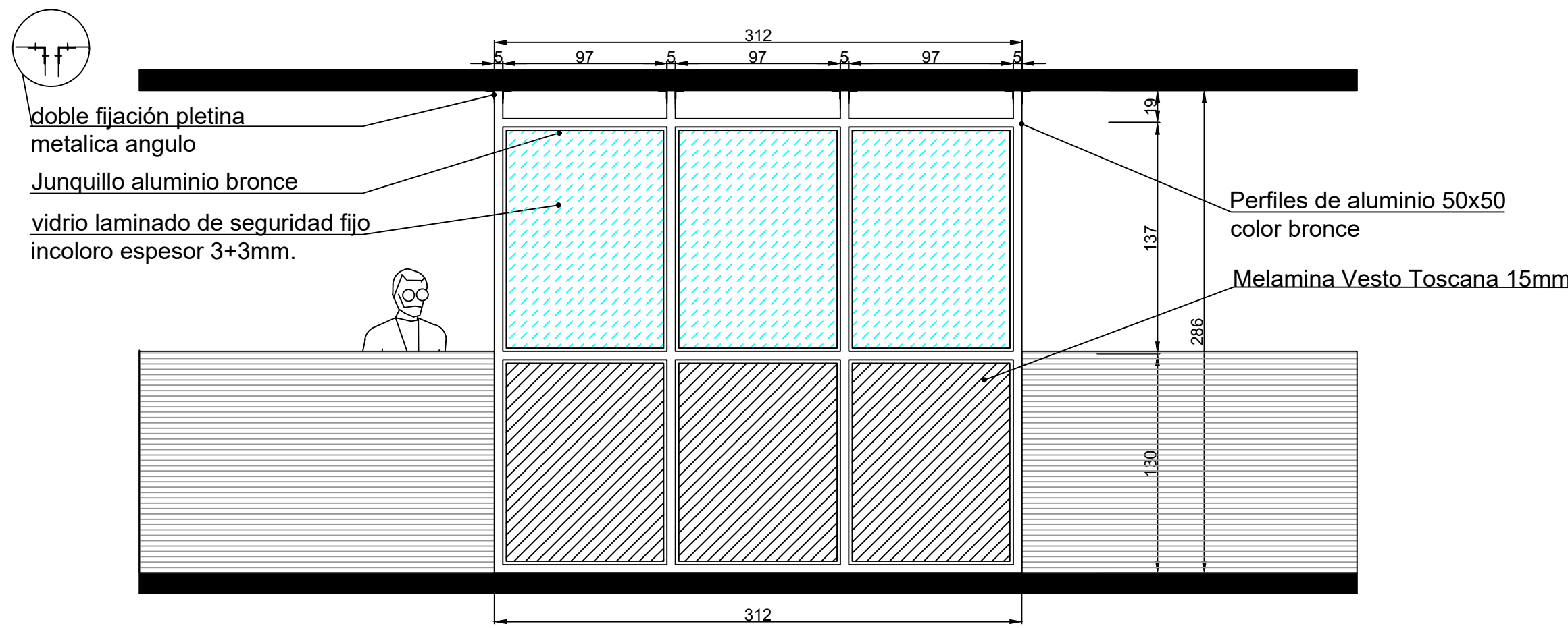
ELEVACIÓN TABIQUE VIDRIADO
